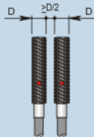
Montaggio affiancato
