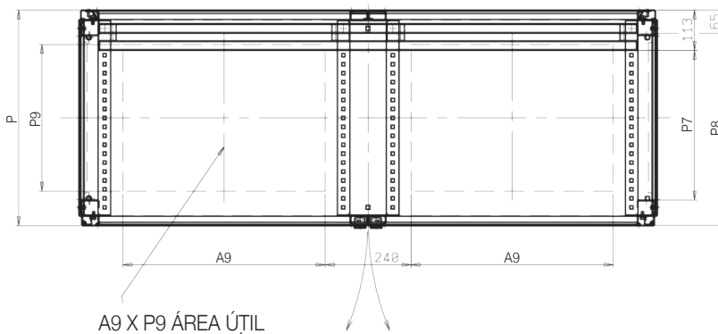
SECCIÓN B-B
