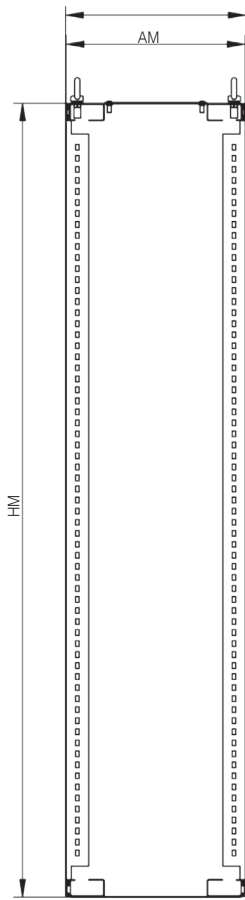
SECCIÓN B-B
