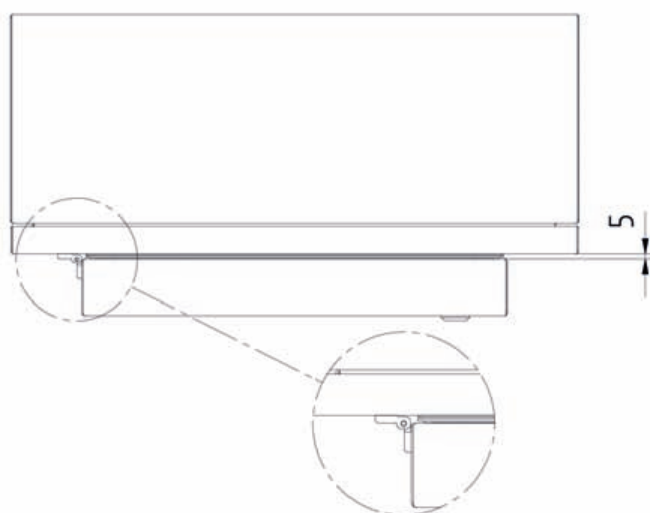
MONTAJE DE BISAGRAS CON APERTURA PUERTA DE PROTECCIÓN A 90°
