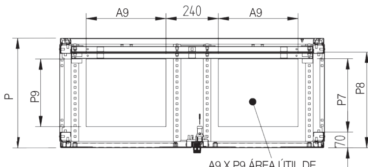
SECCIÓN B-B
