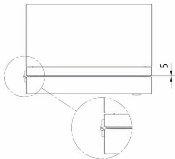
MONTAJE DE BISAGRAS CON APERTURA PUERTA DE PROTECCIÓN A 180° (se debe comprobar en función de la aplicación)
